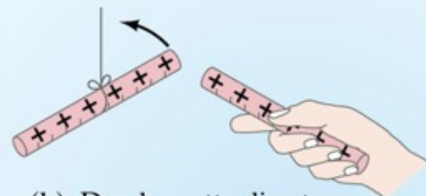
(b) Due barrette di vetro cariche si respingono
