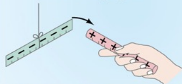
(c) Una barretta di vetro carica attrae un righello di plastica carico
