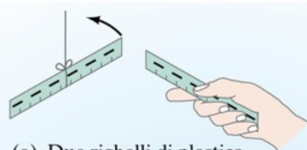
(a) Due righelli di plastica carichi si respingono
